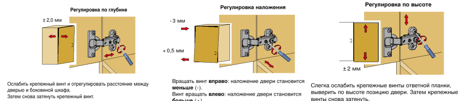
Рис.4 Схема установки петель
