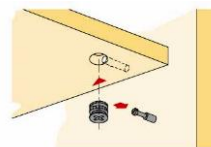
Рис.2 Схема установки эксцентрика
