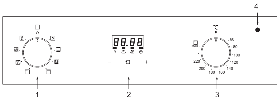
Рис. 1. Панель управления
