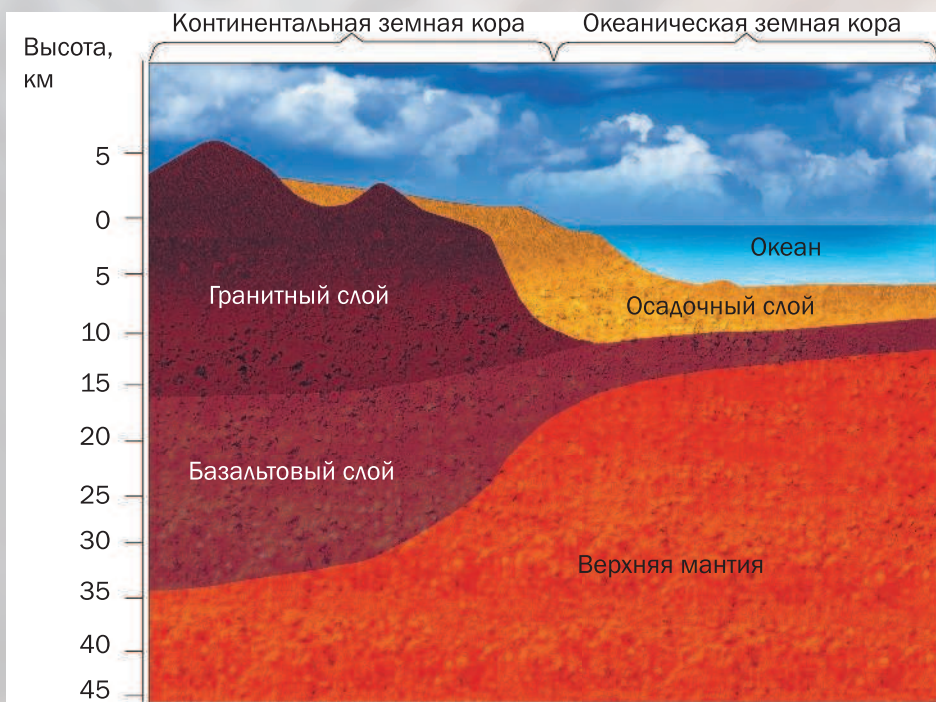
Строение земной коры.
