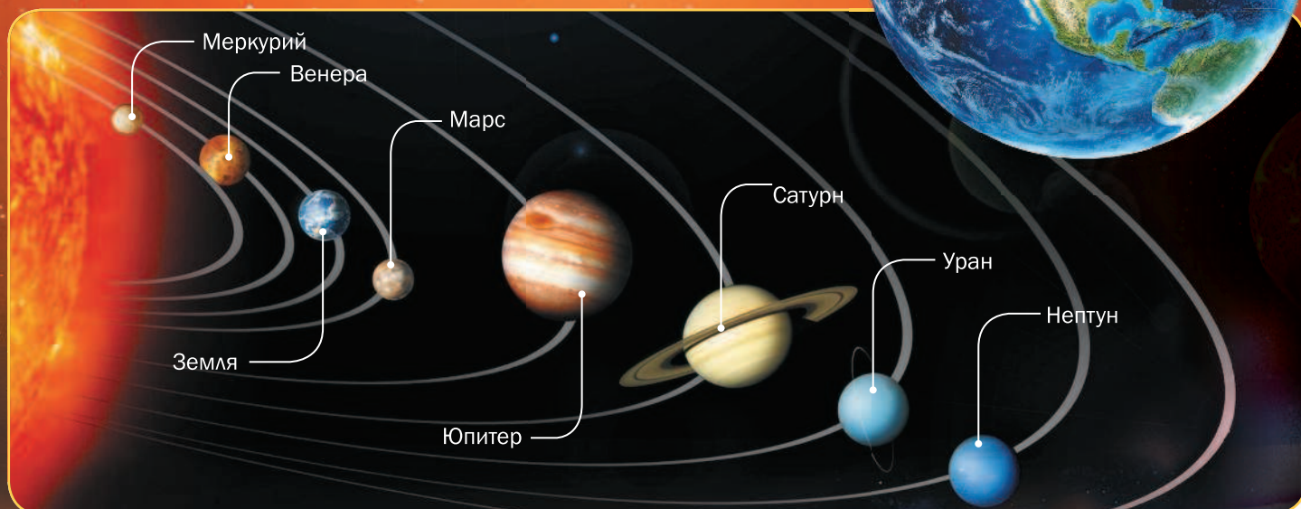
Порядок расположения орбит планет Солнечной системы.
