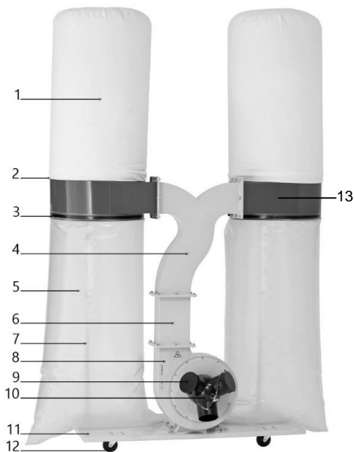
Рисунок 1. Основные элементы вытяжки
