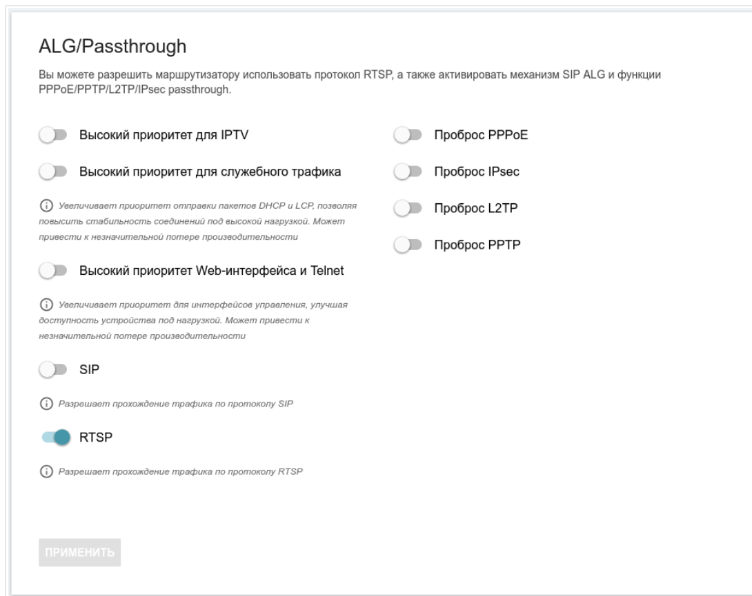
Рисунок 119. Страница Функции / Дополнительно / ALG/Passthrough .
