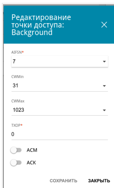
Рисунок 96. Окно для изменения параметров функции WMM.
