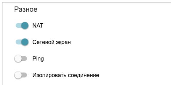
Рисунок 58. Страница добавления соединения типа PPPoE. Раздел Разное.
