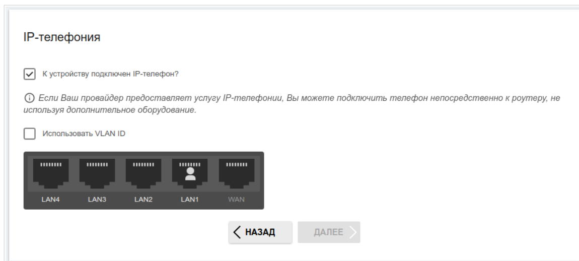
Рисунок 42. Страница выбора LAN-порта для подключения VoIP-телефона.
