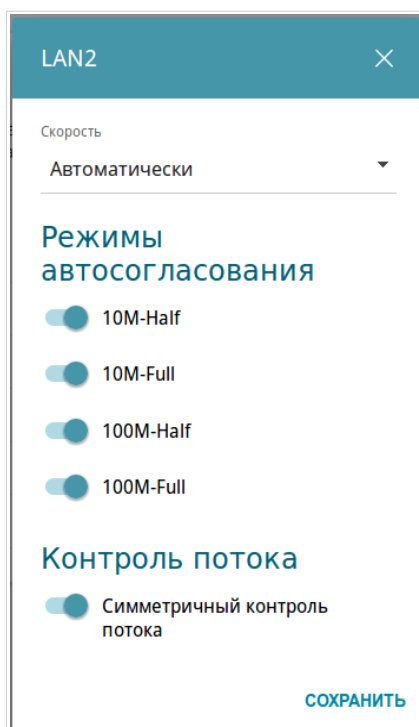
Рисунок 116. Окно изменения настроек порта маршрутизатора.
