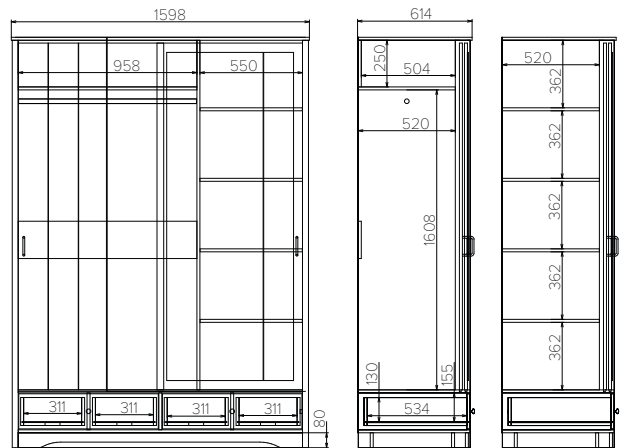
Шкаф купе №2: 1600-600-2200 мм
