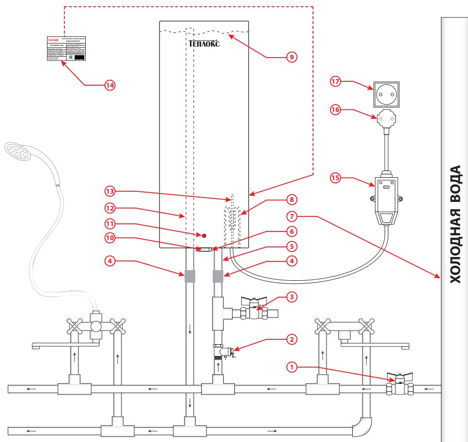
Рис. 1 Общая схема подключения
