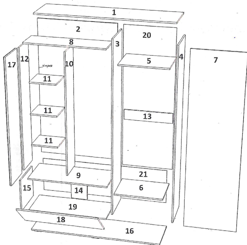
Схема сборки
