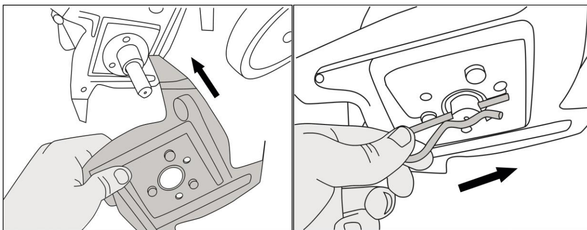
Рис. 5. Установка фрез
