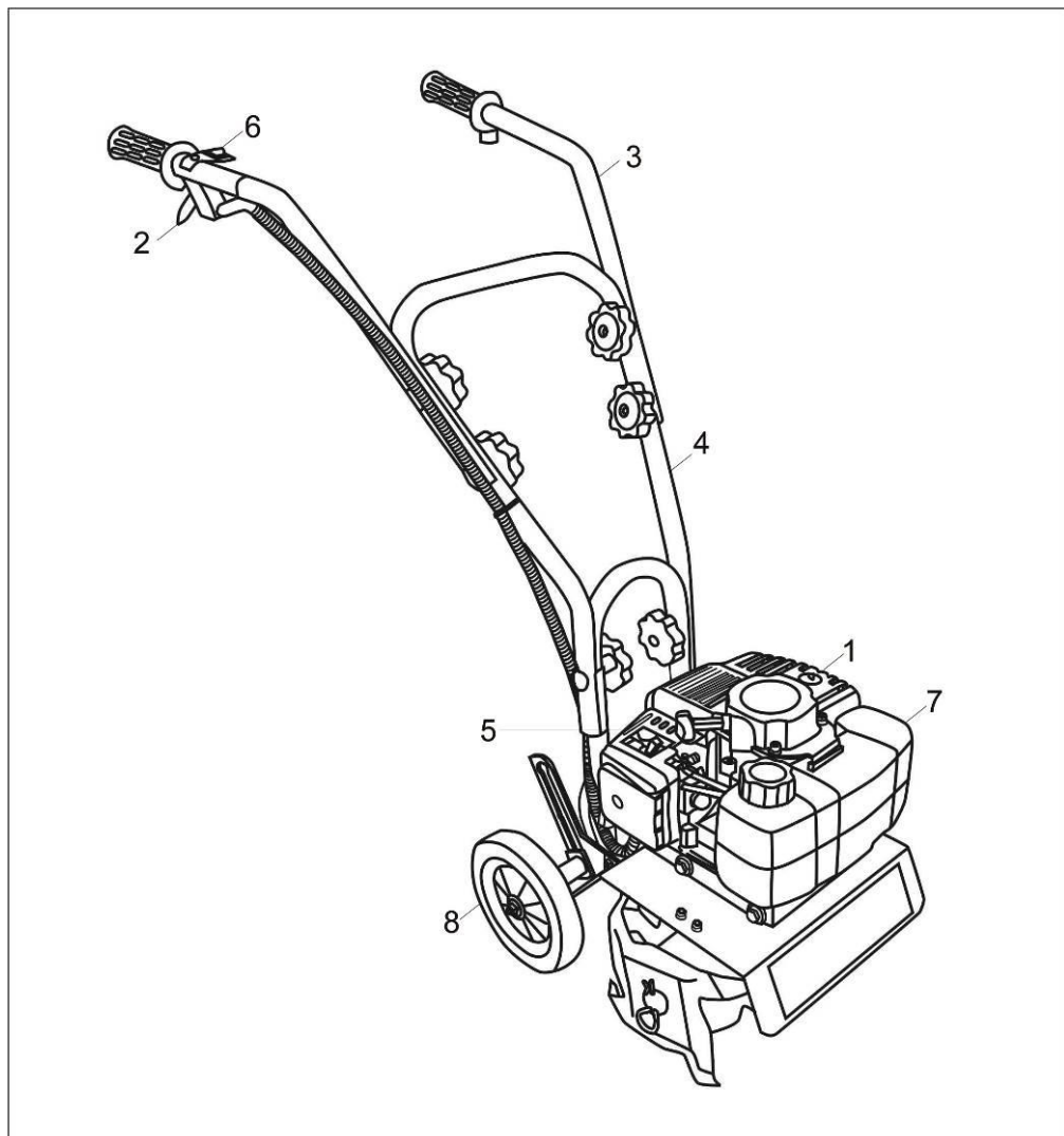
Рис. 1. Основные узлы устройства
