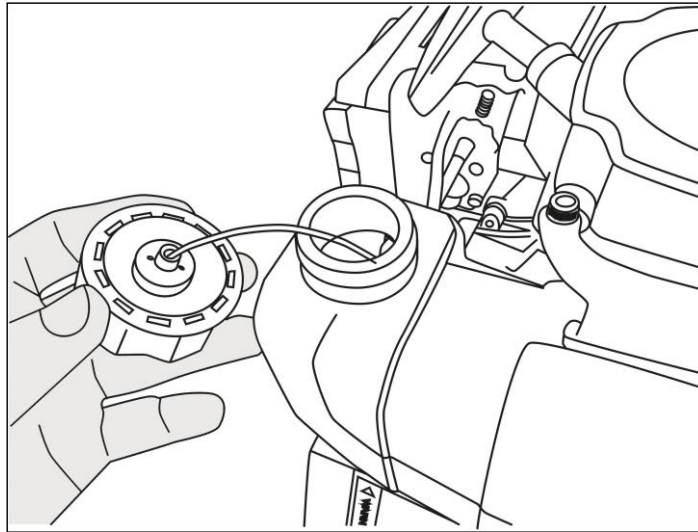
Рис.11. Откручивание крышки
