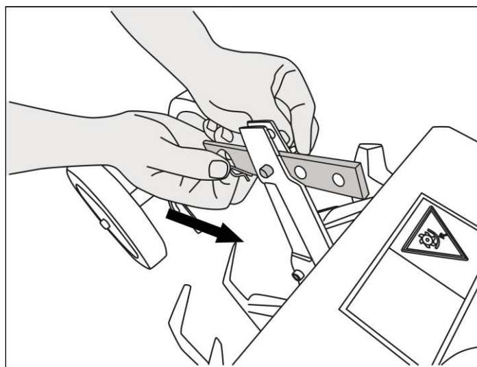
Рис. 6. Установка сошника
