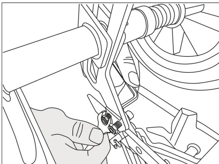
Рис. 7. Фиксация кронштейна с колесами
