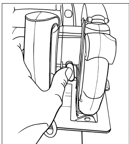
Рис.4 Ослабление фиксатора
