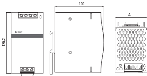
Рис. 3 Габаритные размеры блока питания DR-75W-12, DR-120W-12.
