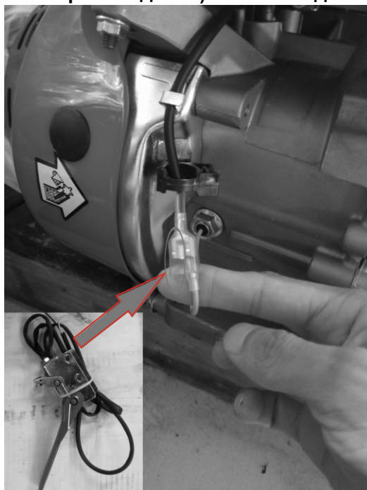
Схема подключения ручки(либо кнопки для некоторых моделей)остановки двигателя
