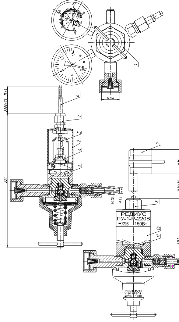
Рис. 2. Регулятор расхода газа баллонный одноступенчатый крупногабаритный с подогревателем У-30-КР2П (сверху) и У-30-КР2П1 (220В) (снизу):
