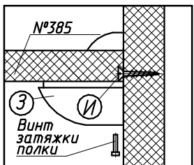
Крепление для полок (комплект №40)
