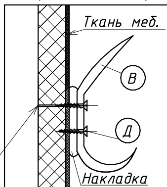
Крепление крючка (комплект №30)
