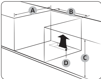
Шафа під умивальником (мм)
