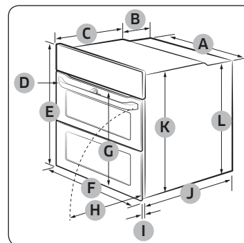
Пеш (мм)
