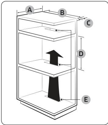
Вбудована шафа (мм)
