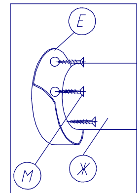
Крепление штанги (комплект №6)
