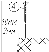
Крепление винта саморезного (комплект №19)
