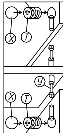
Крепление стяжки эксцентриковой (комплект №45)
