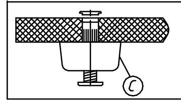
Крепление опоры (комплект №26)
