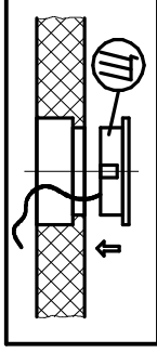
Крепление задней стенки (комплект №10)
