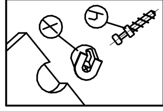
Крепление стяжки эксцентриковой (комплект №45А)
