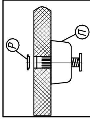
Крепление опоры (комплект №26)
