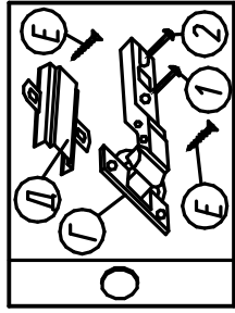
Крепление петель (комплект №4)
