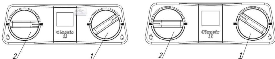
а) Ручки регулировки расхода воды 1 и расхода газа 2 в положении “Минимальный расход” б) Ручки регулировки расхода воды 1 и расхода газа 2 в положении “Максимальный расход”
