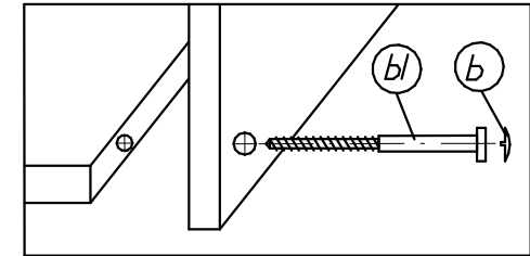
Крепление винта саморезного (комплект №19)
