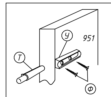
Крепление K-PUSH (комплект №92)
