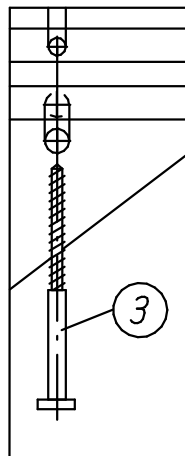
Крепление винта саморезного (комплект №19)
