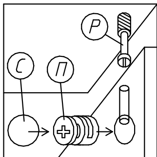
Крепление стяжки эксцентриковой (комплект №45)
