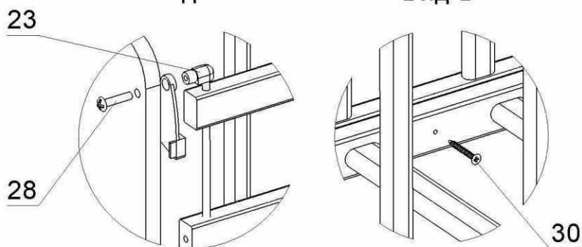
Вид Б
