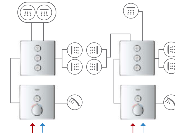
КОМБИНАЦИЯ (ТЕРМОСТАТ)
