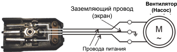
Рис. Подсоединение проводов от вентилятора/насоса к вилке
