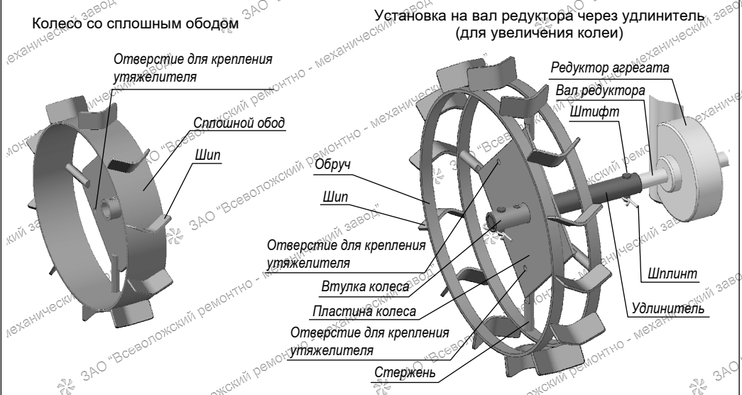
Рис. 1 Варианты установки колёс на агрегат
