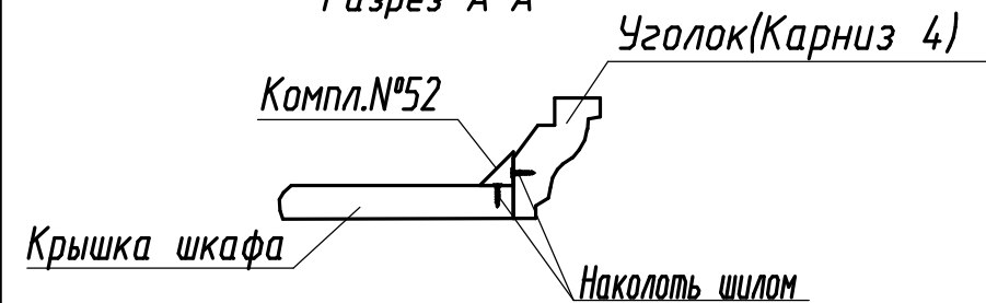
Разрез А-А
