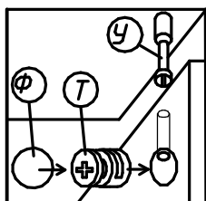
Крепление стяжки эксцентриковой (комплект №45)
