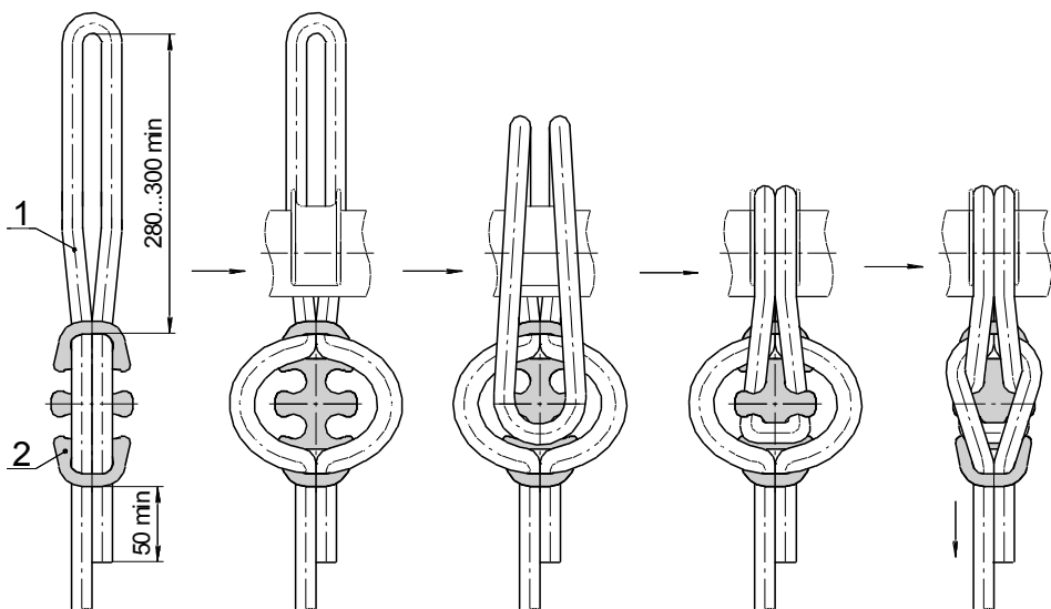
Рис.2. Схема безузлового крепления фиксатора на шнуре
