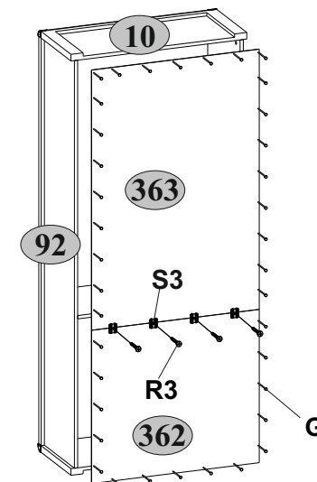
Шкаф с витриной 2V2D1S «MAGELLAN» Cabinet-showcase 2V2D1S Szafla-witryna 2V2D1S
