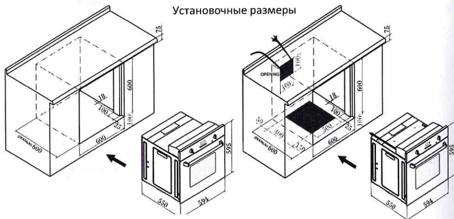
Электрическая духовка
