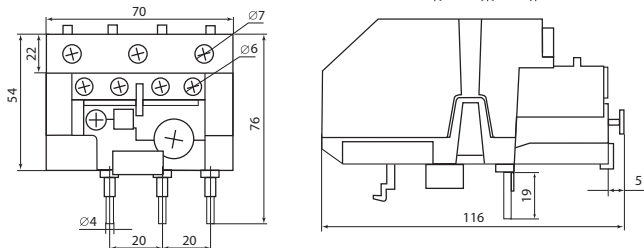
Рисунок 4. Габаритные и установочные размеры реле PTH-3353...PTH-3365, мм
