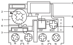
Рисунок 6. Передняя панель реле
