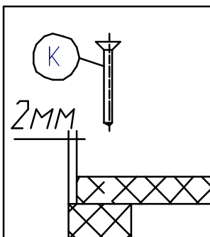
Крепление подвески (комплект №20)
