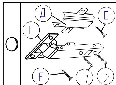
Крепление петли (комплект №4)
