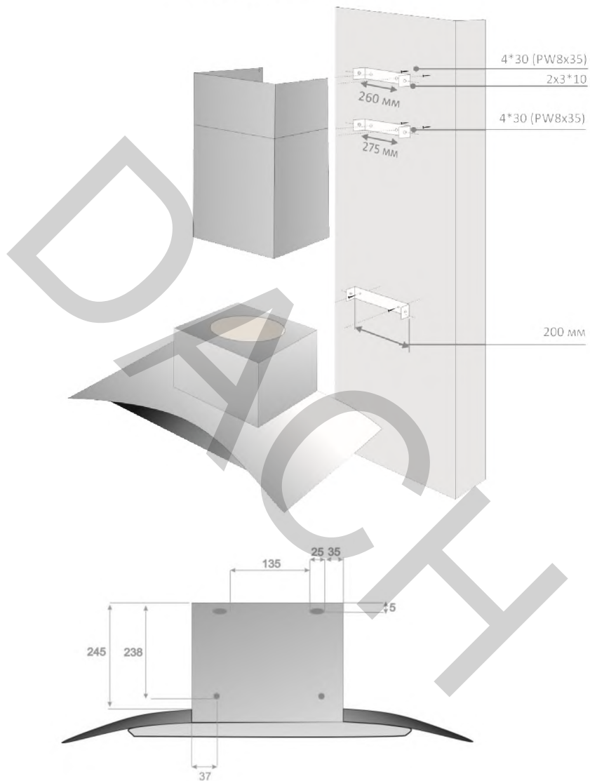
Мал. 8 Схема мантажу выцяжкі
