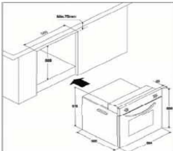
Электрическая духовка
