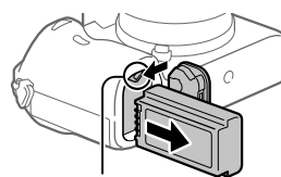
Рычаг блокировки
