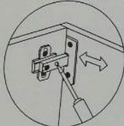
установка дверей
