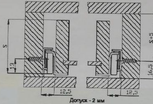
Схема установки направляющих ящика
