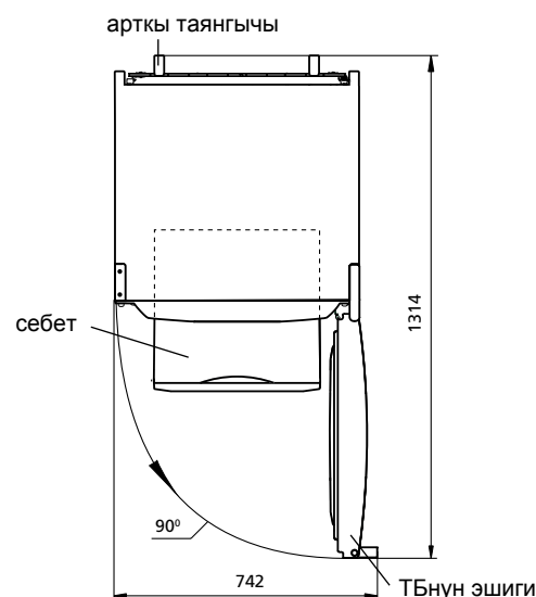
2-сүрөт — Муздаткыч (жогору жагынан көрүнгөн көрүнүшү)
