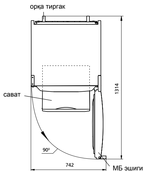
2-расм — Совутқич (уст қисми билан кўриниши)
