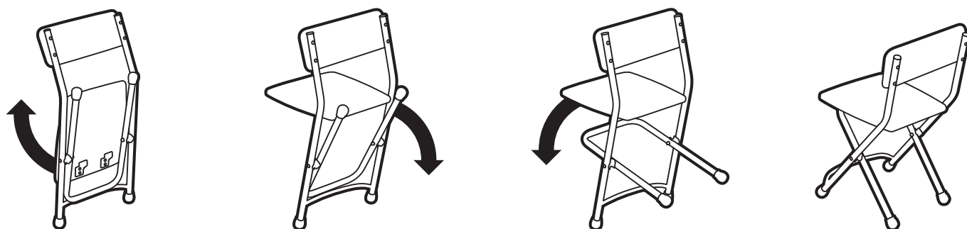
(рис. 5) Схема раскладывания стула с мягкой обивкой
