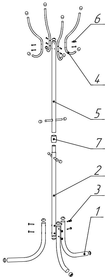
Рис. 1 Схема сборки
