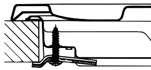
Монтаж крюка для опорных брусков H=30 мм
