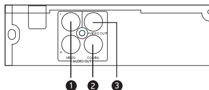
Задняя панель
