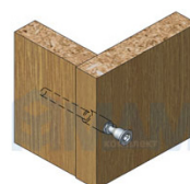
Евровинт 7 * 50
