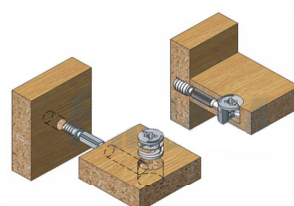
Стяжка эксцентриковая
