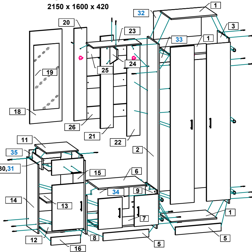
Комплектовочная ведомость на детали
