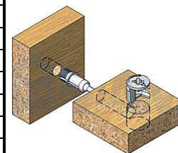
Соединение деталей эксцентриковыми стяжками
