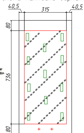
Схема наклейки зеркала
