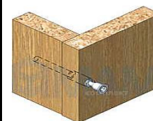
Соединение деталей евровинтами
