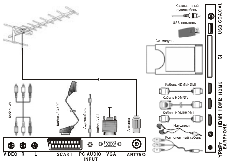
Рисунок 5 – Типовая схема подключения внешних устройств
