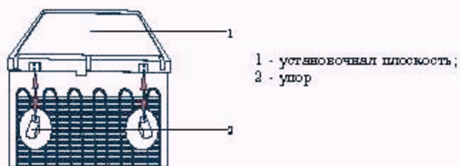
Рисунок Б.1а - Схема крепления упоров к плоскости установочной (сервировочной)
