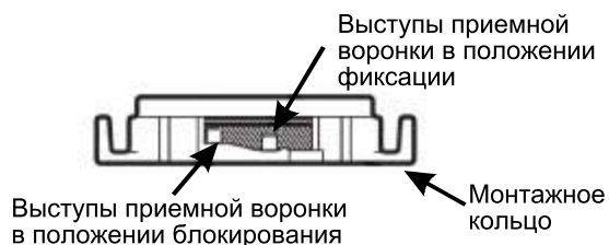
Фиксация детали
