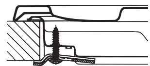
Konsude asukoht aluspinnal H=30mm
