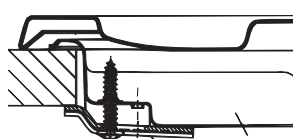
Nostiprināšanas pozīcija galdā virsmām ar H=20mm
