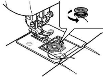
Крышка челнока
