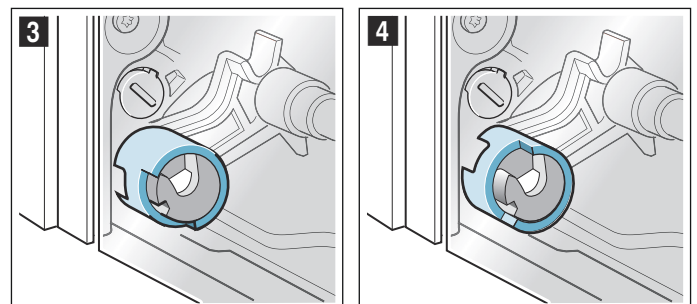
Фиксатор петли закрыт (рис. 3 ) Фиксатор петли открыт (рис. 4 )
